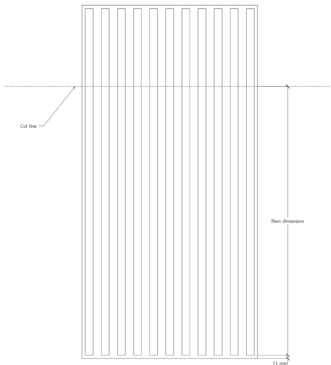
Figure 4. Coupe perpendiculaire aux lames principales sur une tuile ELEMENT.
