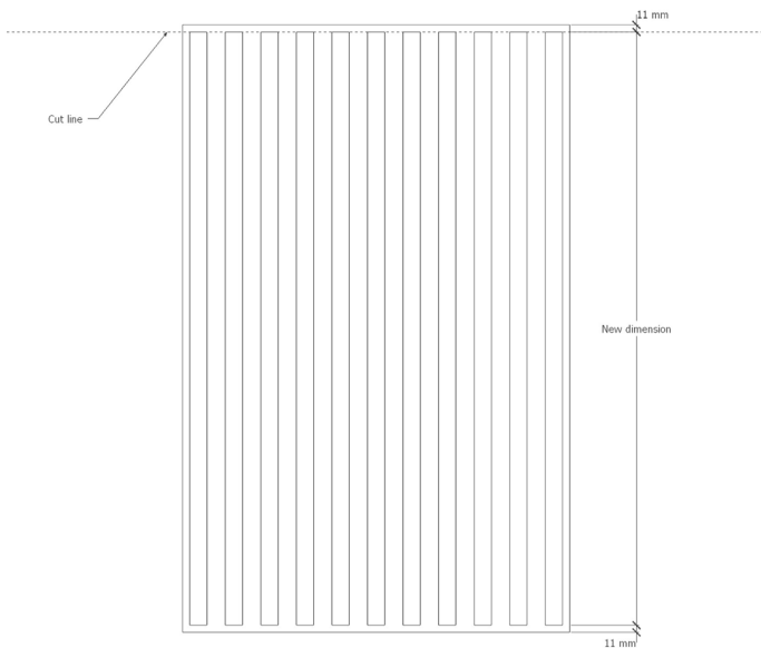
Figure 5. Positionnement de la nouvelle lame de soutien sur une tuile ELEMENT.
