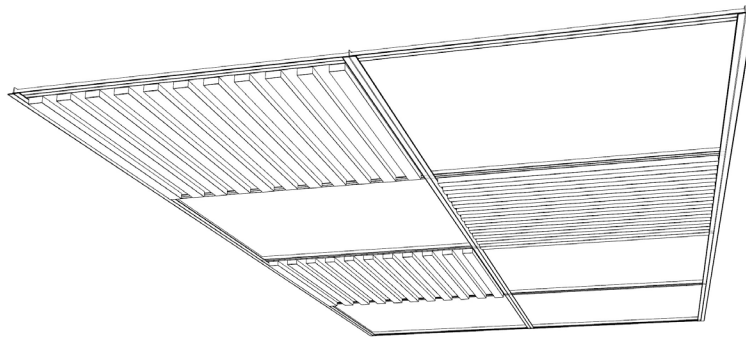
Figure 2. Installation des tuiles HARMONY, avec une trame de 24po x 24po.
