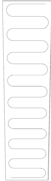
Figure 2. Fixation chimique du panneau HARMONY FLEX avec de l'adhésif à construction.
