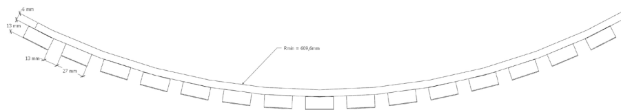
Figure 5. Rayon de courbure maximal de 24po du panneau HARMONY FLEX.
