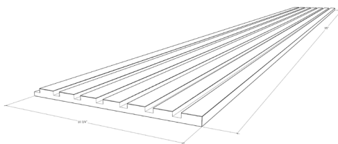
Isométrie - Panneau STRATA avec cotations
