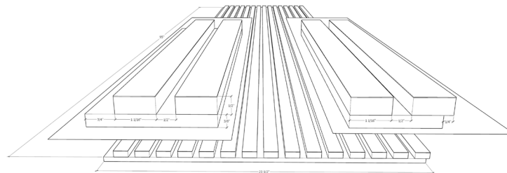
Isométrie- Panneau HARMONY avec cotations
