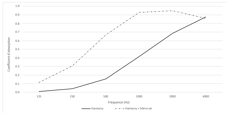
Rendement acoustique de la collection HARMONY
